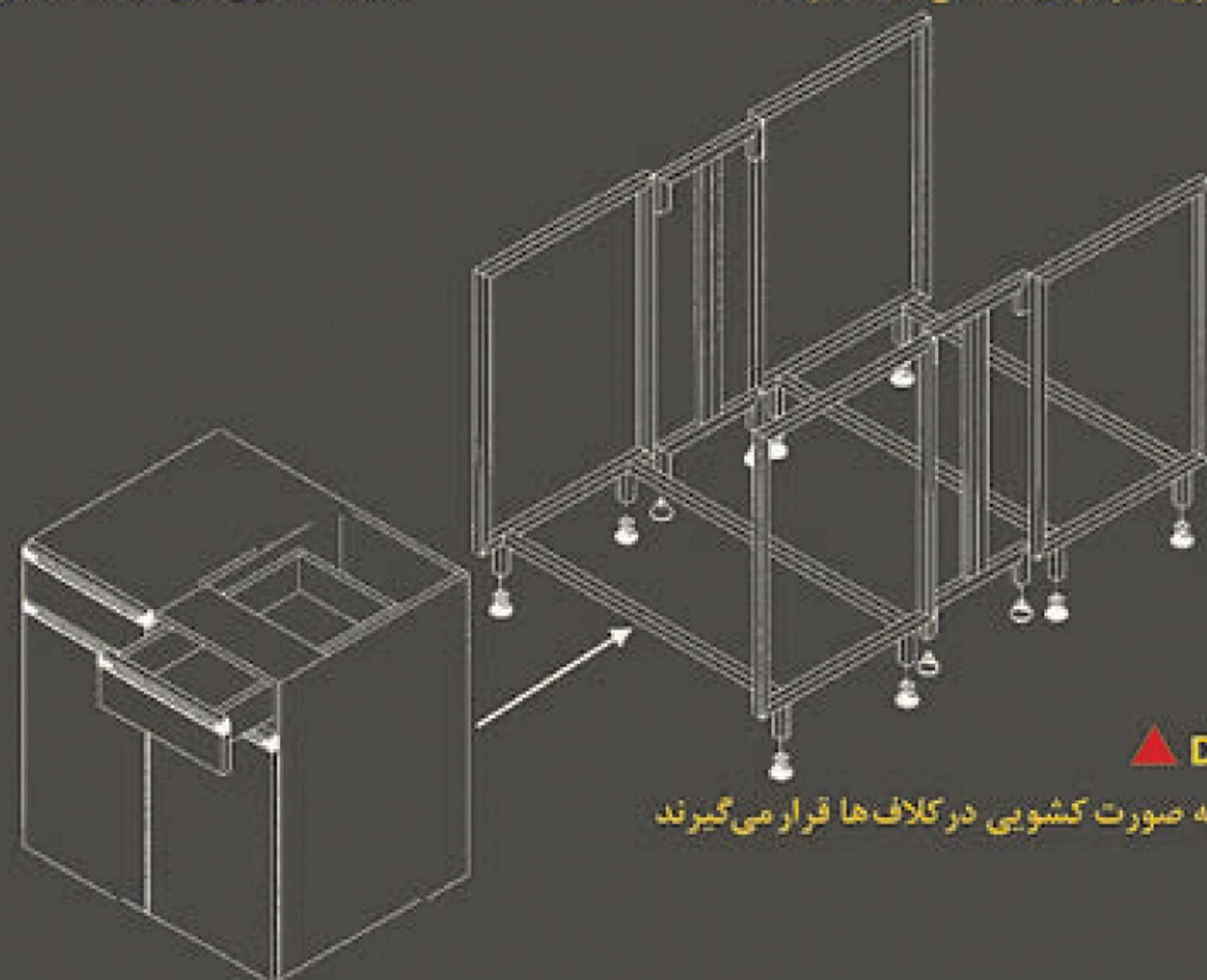
▲ Detail - 2 اسکلت فلزی میز آزمایشگاهی (دو طرفه)
